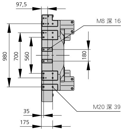
机械手系统的固定 | C
