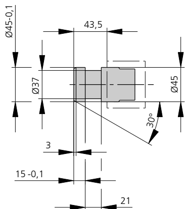
顶针杆 | X
