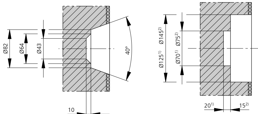
模具镗孔（需要时）| Y
